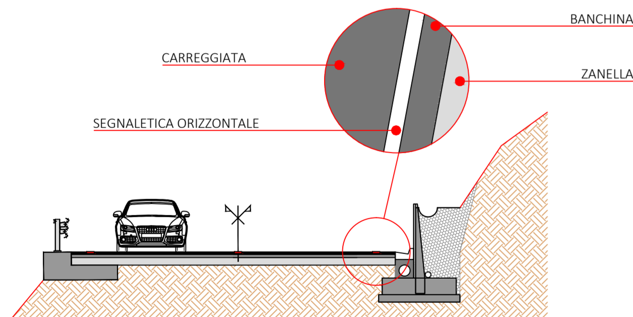
PARTICOLARE SEGNALETICA STRADALE ORIZZONTALE
