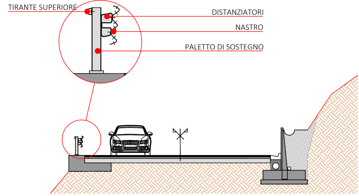
PARTICOLARE SISTEMAZIONE STRADALE
