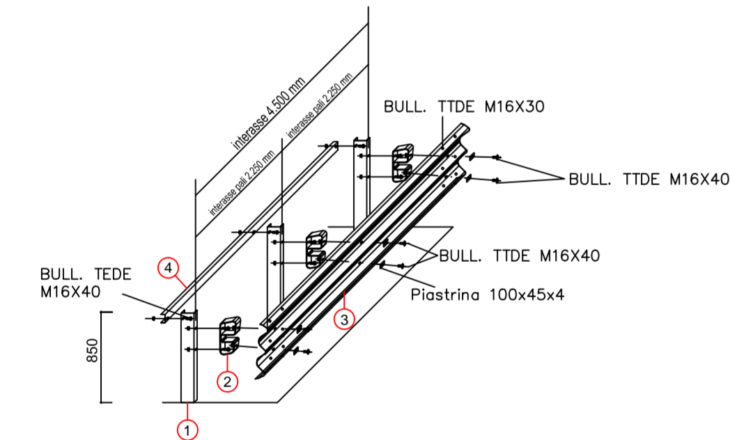
BARRIERA STRADALE TIPO H2
