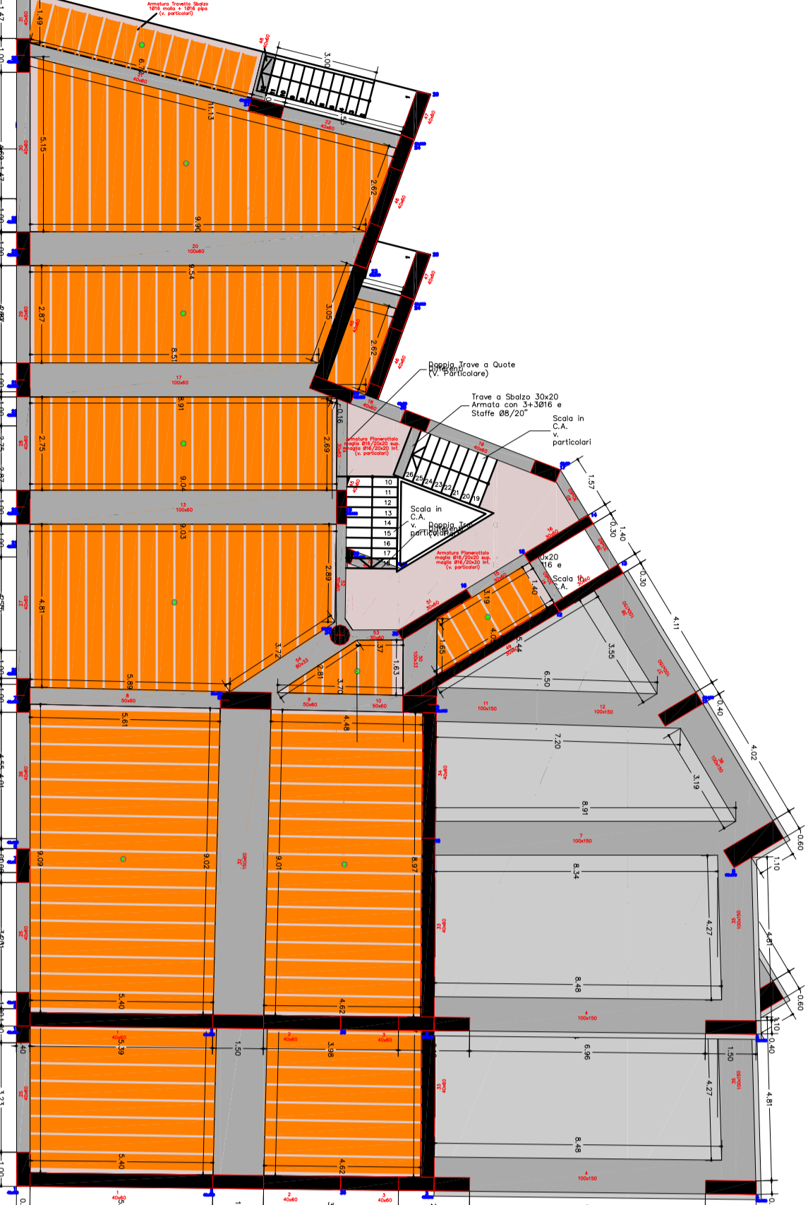
Piano di livello 1 - Quoto 4.93 m.
