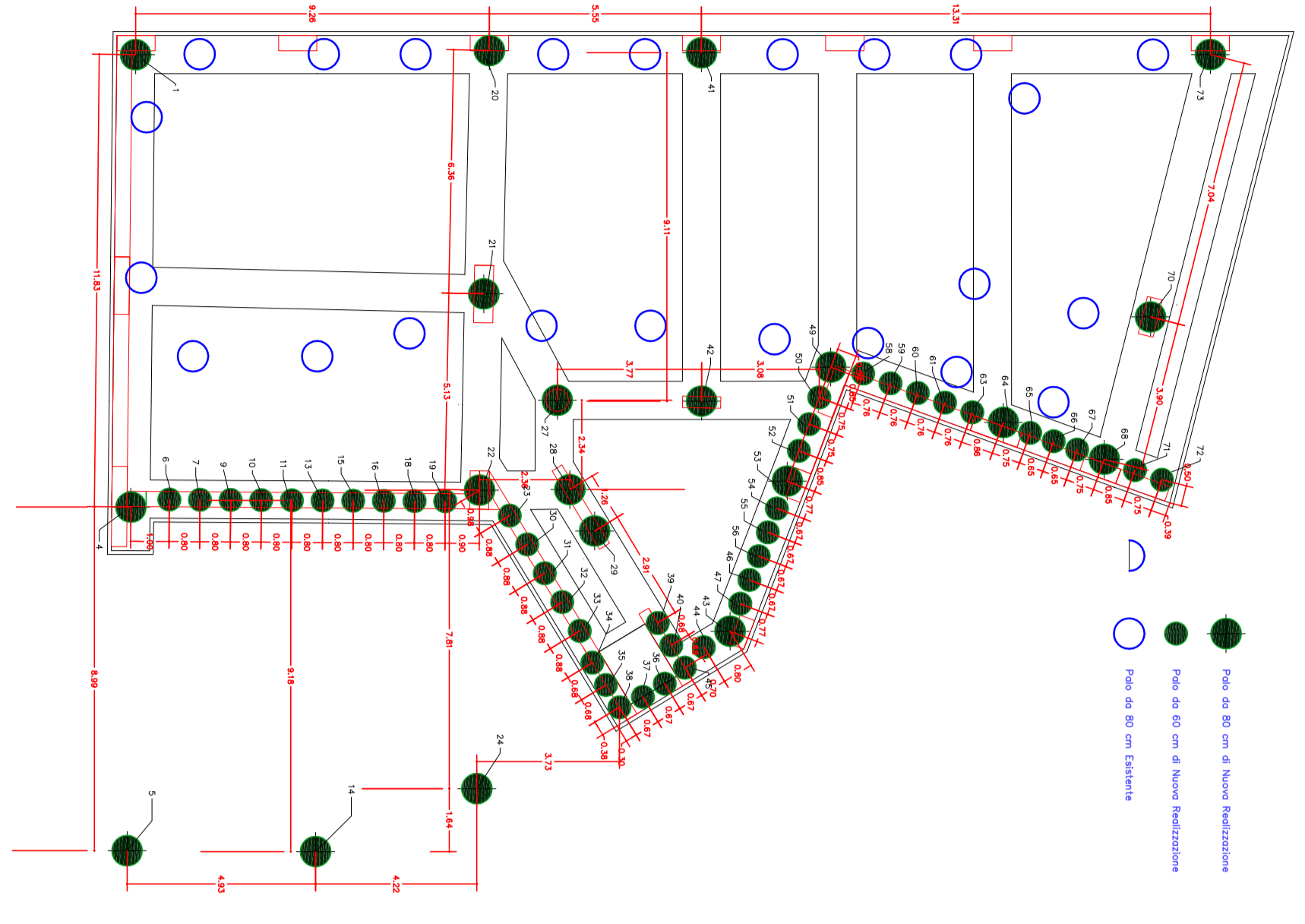
PIANTA PIANO FONDAZIONI E SCHEMA PALI
